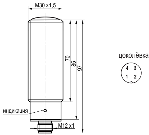
Габаритный чертёж.
